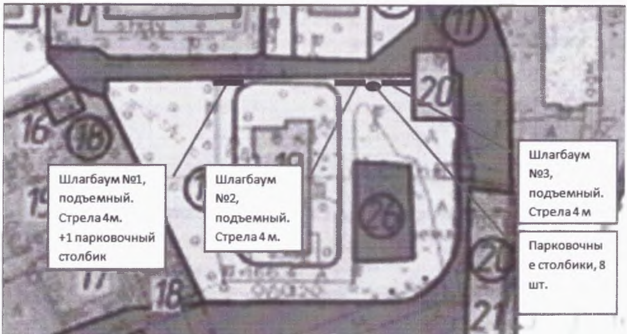
Схема размещения шлагбаумов.
